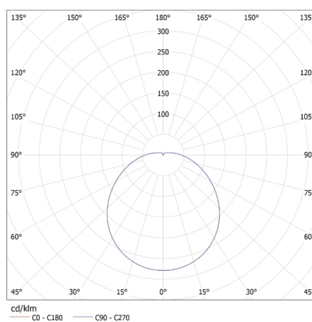
MILED0 (kat 31099) CORSO LED N 12-NW-SE / LDC (Polar)
