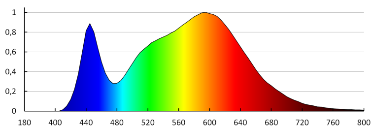
MILED0 (kat 31099) CORSO LED N 12-NW-SE / LDC (Polar)
