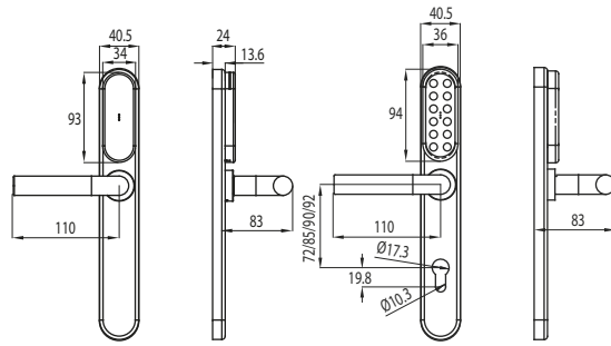
Ext. Escutcheon (LS1)
